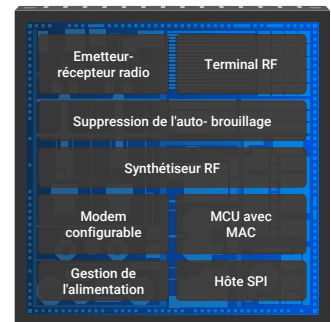
Puces pour lecteur de la série Impinj E700
