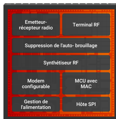
Puces pour lecteur de la série Impinj E500
