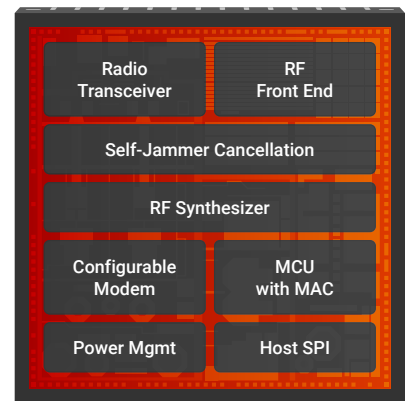
Impinj E510 Reader Chip
