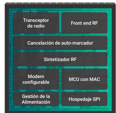
Chips de lectores de la serie de Impinj E300
